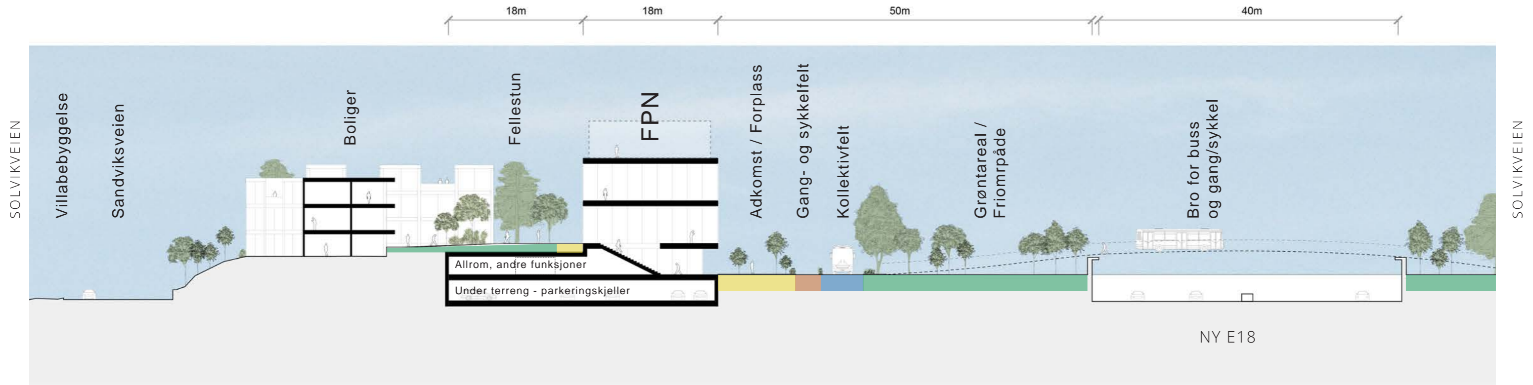
TVERRSNITT
